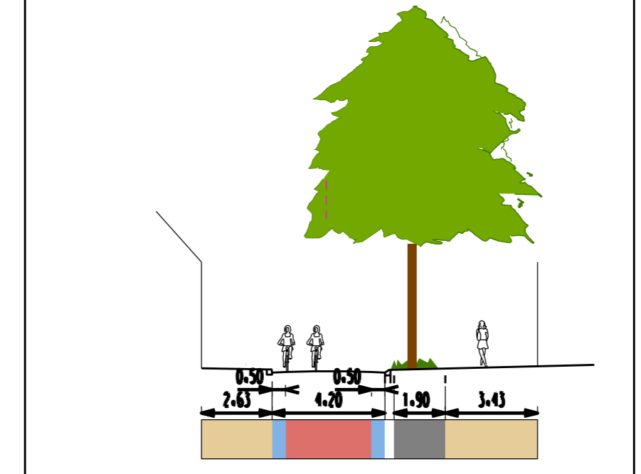
Dwarsprofiel Dolmanstraat tussen nr 52 en 54
