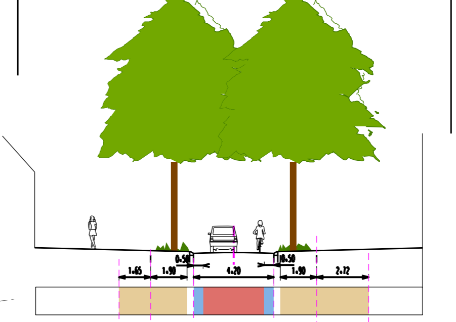
Dwarsprofiel Dolmanstraat tussen nr 52 en 54
