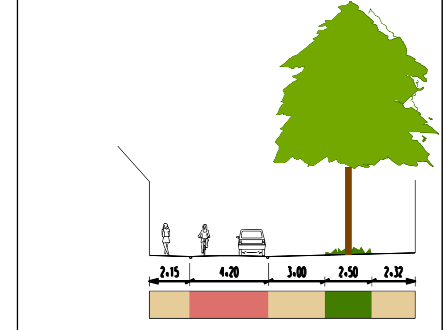
Dwarsprofiel Dolmanstraat t.h.v. kerk
