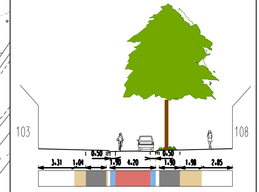
Dwarsprofiel Populierweg t.h.v. huisnr 108
